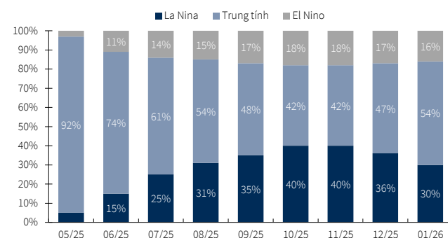
Biểu đồ 7. Xác suất các pha thời tiết trong 2025
